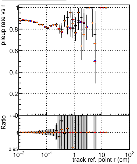
■ DQM original lowpt ● DQM newbranch lowpt ▲ DQM original lowpt pless × DQM newbranch lowpt pless
