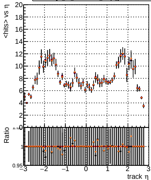
mean hit — DQM TT original lowpt — DQM TT newbranch lowpt — DQM TT original lowpt pLess — DQM TT newbranch lowpt pLess
