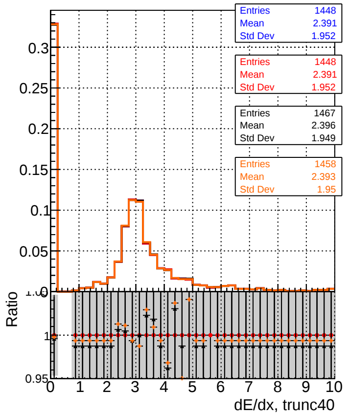
dE/dx estimator 2
