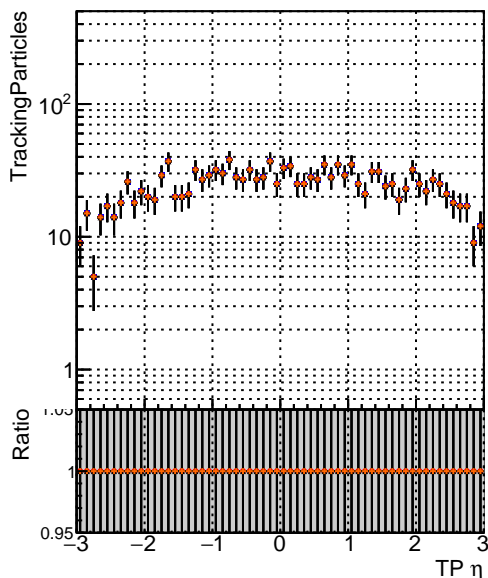
N of sim ● DQM TT newbranch_lowpt ▲ DQM TT original_lowpt_pLess ◆ DQM TT newbranch_lowpt_pLess
