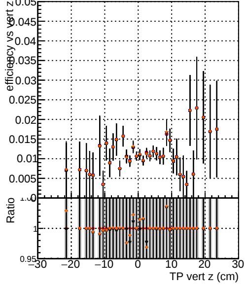
Efficiency vs. TP vert z — DQM TT original_lowpt — DQM TT newbranch_lowpt — DQM TT original_lowpt_pLess — DQM TT newbranch_lowpt_pLess
