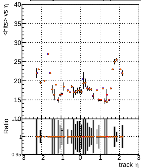
mean hit Legend: — DQM TT original lowpt — DQM TT newbranch lowpt — DQM TT original lowpt pLess — DQM TT newbranch lowpt pLess
