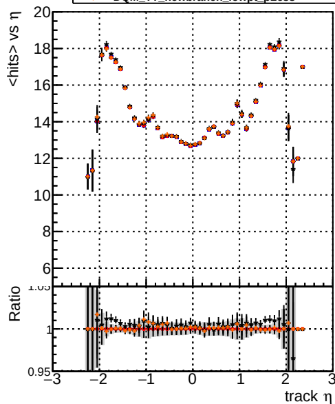
Legend: — DQM TT original_lowpt — DQM TT newbranch_lowpt — DQM TT original_lowpt_pLess — DQM TT newbranch_lowpt_pLess
