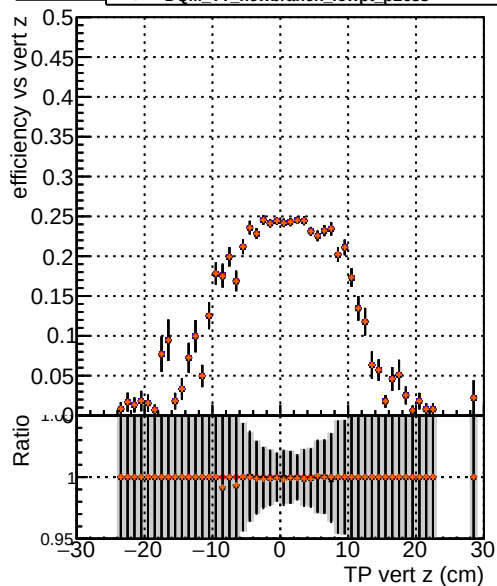
Efficiency vs. sim PV z — DQM TT original_lowpt — DQM TT newbranch_lowpt — DQM TT original_lowpt_pLess — DQM TT newbranch_lowpt_pLess
