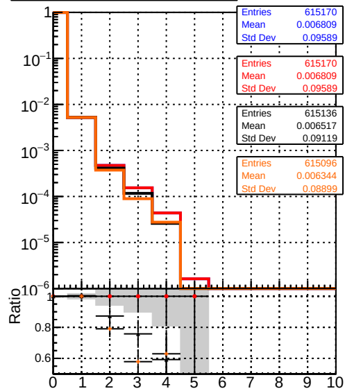
— DQM TT original — DQM TT newbranch — DQM TT original pLess — DQM TT newbranch pLess
