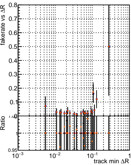
Fake rate vs —●— DQM TT original —●— DQM TT newbranch —●— DQM TT original pLess —●— DQM TT newbranch pLess
