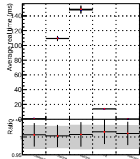
ConvStep
