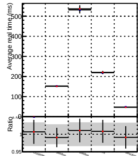
lowPTQuadStep
