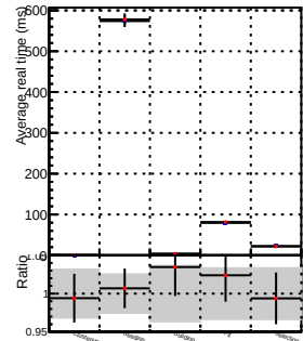
pixelLessStep
