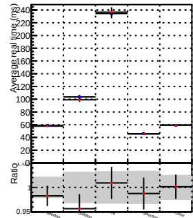
InitialStep
