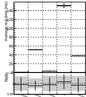
highPTTripletStep
