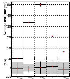
pixelPairStep
