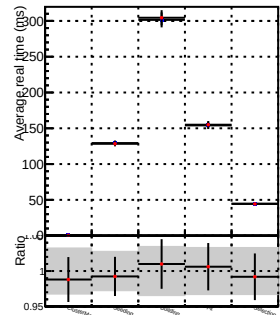
lowPTTripletStep
