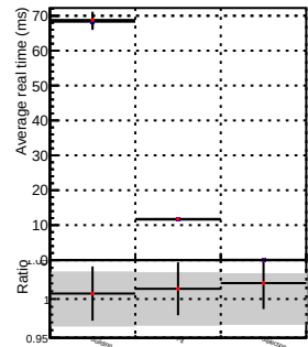
duplicateMerge
