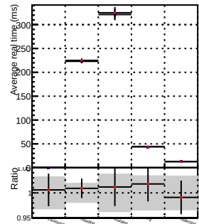
toBecStep
