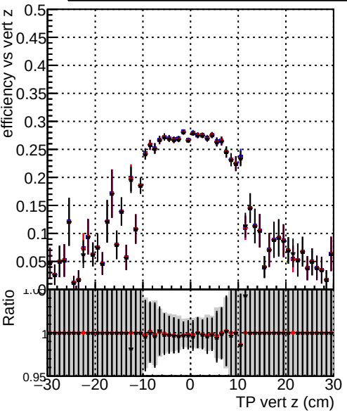
Efficiency vs vert z Legend: DQM_test_CKFFitDefault DQM_test_doubleFit_noOL DQM_test_mkFitFit_noOL
