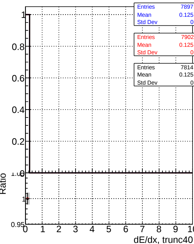
dE/dx estimator 2
