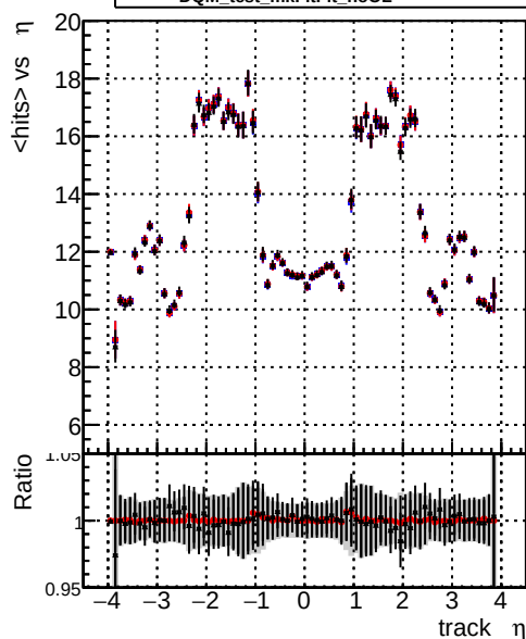
mean hit — DQM_test_CKFFitDefault — DQM_test_doubleFit_noOL — DQM_test_mkFitFit_noOL
