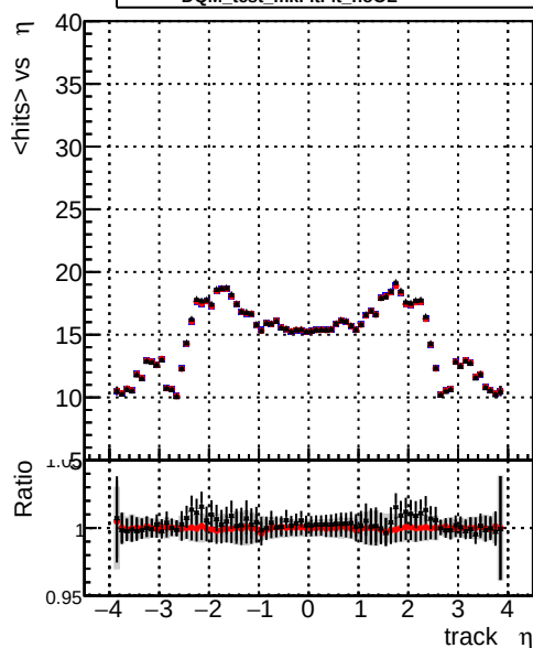
mean hits vs \eta — DQM_test_CKFFitDefault — DQM_test_doubleFit_noOL — DQM_test_mkFitFit_noOL
