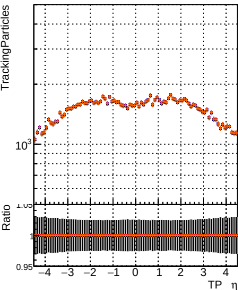
—●— DQM_test_CKFFitDefault —●— DQM_test_mkFitFit —●— DQM_test_mkFitFit_noOL —●— DQM_test_mkFitNOFit_retest
