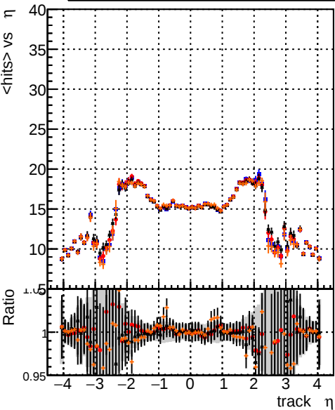
mean hits vs \eta DQM_test_CKFitDefault DQM_test_mkFitFit DQM_test_mkFitFit_noOL DQM_test_mkFitNOFit_retest
