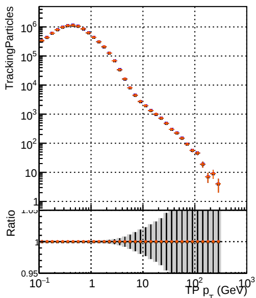
—•— DQM_test_CKFitDefault —•— DQM_test_mkFitFit —•— DQM_test_mkFitFit_noOL —•— DQM_test_mkFitNOFit_retest
