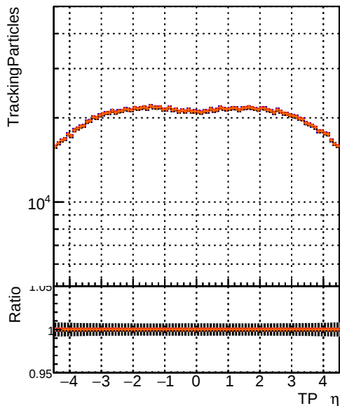
—•— DQM_test_CKFitDefault —•— DQM_test_mkFitFit —•— DQM_test_mkFitFit_noOL —•— DQM_test_mkFitNOFit_retest
