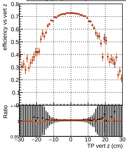
Efficiency vs vert z — DQM_test_CKFfitDefault — DQM_test_mkFitFit — DQM_test_mkFitFit_retest — DQM_test_mkFitNOFit_retest
