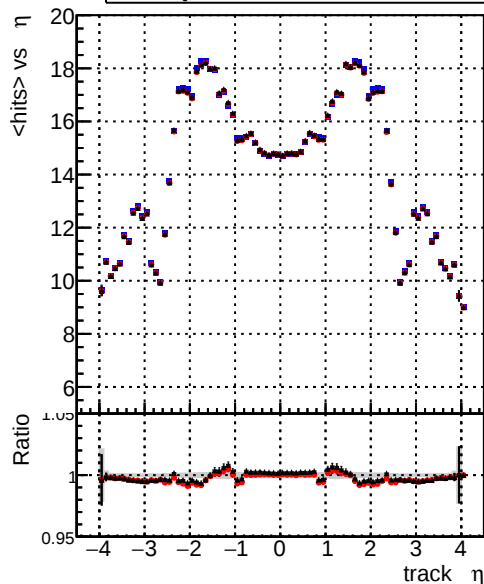
— DQM_test_CKFFitDefault — DQM_test_doubleFit — DQM_test_mkFitFit_newOL3 mean hits
