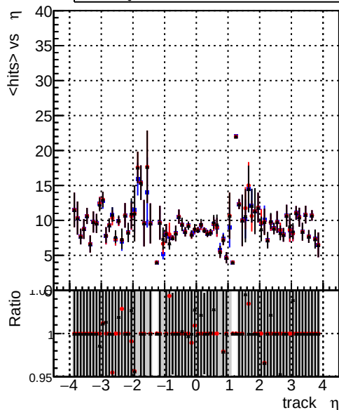
mean hits vs \eta — DQM_test_CKFFitDefault — DQM_test_doubleFit — DQM_test_mkFitFit_newOL3
