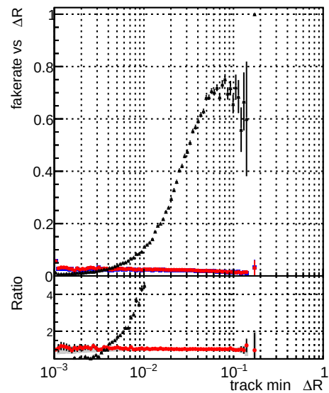
— DQM test CKFitDefault — DQM test doubleFit — DQM test mkFitFit_newOL3
