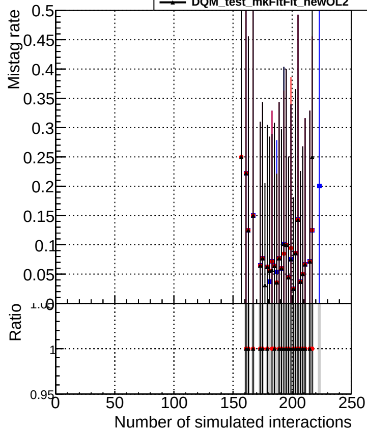
DQM_test_CKFFitDefault DQM_test_doubleFit DQM_test_mkFitFit_newOL2
