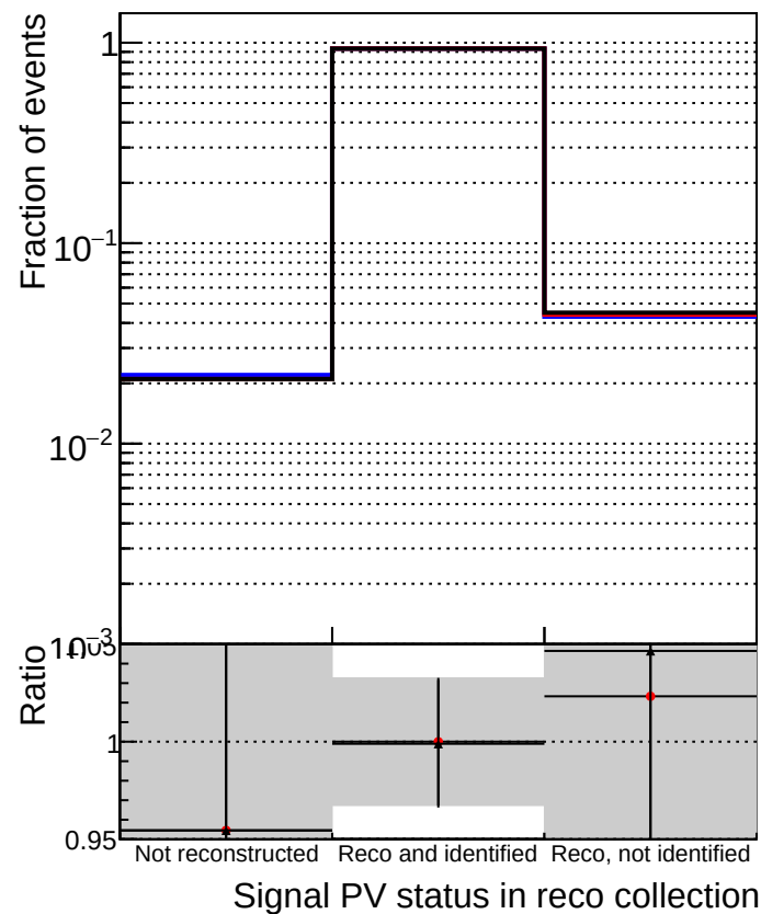
DQM_test_CKFFitDefault DQM_test_doubleFit DQM_test_mkFitFit_newOL2
