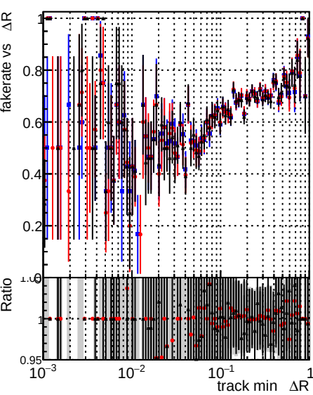
Legend: DQM test CKFitDefault (blue), DQM test doubleFit (red), DQM test mkFitFit_newOL2 (black)
