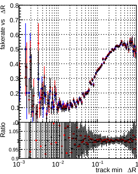
Legend: \bullet DQM_test_CKFFitDefault \bullet DQM_test_doubleFit \bullet DQM_test_mkFitFit_newOL2
