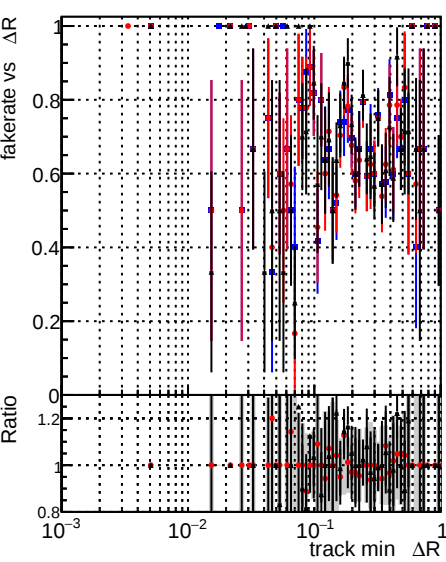
Fake rate vs \Delta R(\text{track, jet}) DQM_test_CKFFitDefault DQM_test_doubleFit DQM_test_mkFitFit_newOL2
