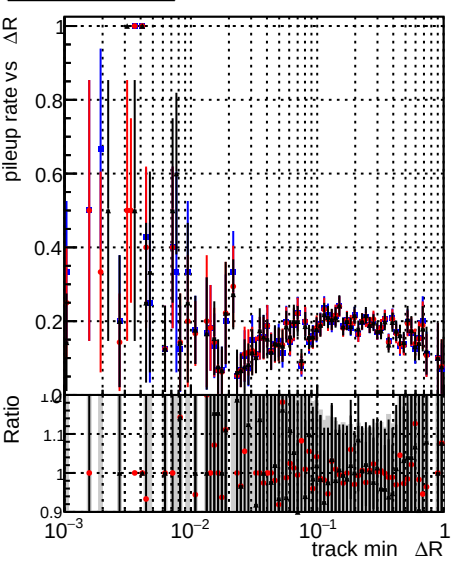
Legend: DQM test CKFitDefault (blue), DQM test doubleFit (red), DQM test mkFitFit_newOL2 (black)
