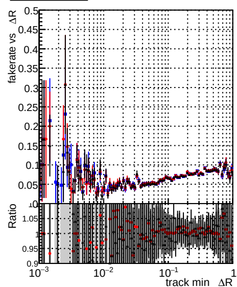
— DQM test CKFitDefault — DQM test doubleFit — DQM test mkFitFit_newOL2
