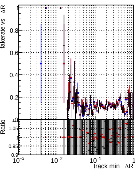
Fake rate vs \Delta R(\text{track, jet}) DQM test CKFitDefault DQM test doubleFit DQM test mkFitFit_newOL2
