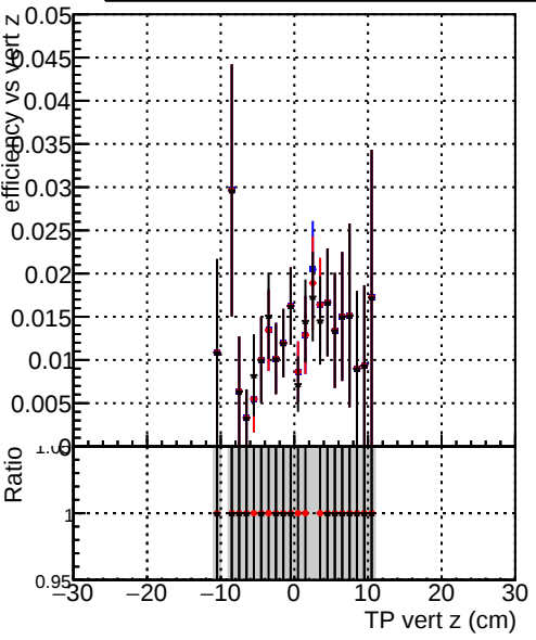
Efficiency vs TP vert z (cm) Legend: DQM_test_CKFFitDefault DQM_test_doubleFit DQM_test_mkFitFit_newOL2
