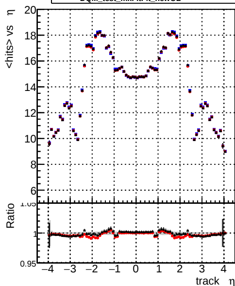
mean hits — DQM_test_CKFFitDefault — DQM_test_doubleFit — DQM_test_mkFitFit_newOL
