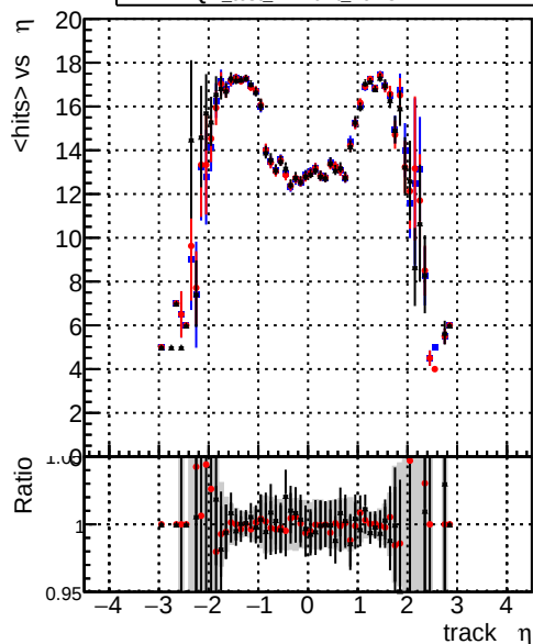
— DQM_test_CKFFitDefault — DQM_test_doubleFit — DQM_test_mkFitFit_newOL mean hits
