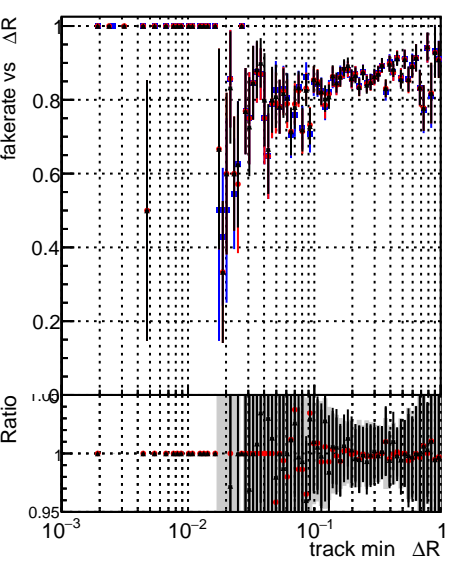
■ DQM_test_CKFFitDefault ● DQM_test_doubleFit ▲ DQM_test_mkFitFit_newOL
