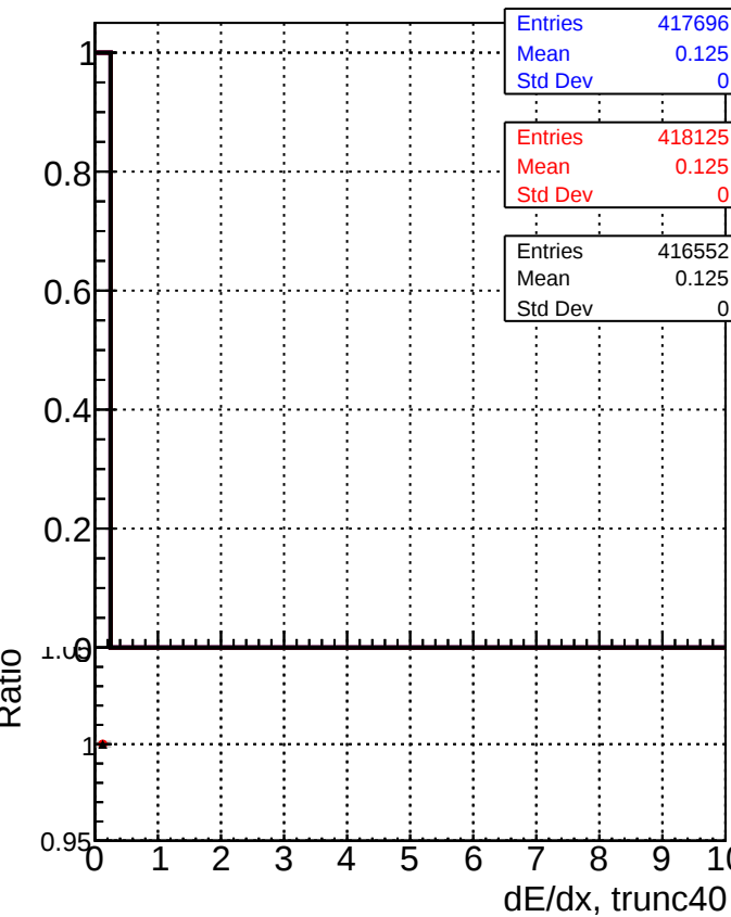
dE/dx estimator 2
