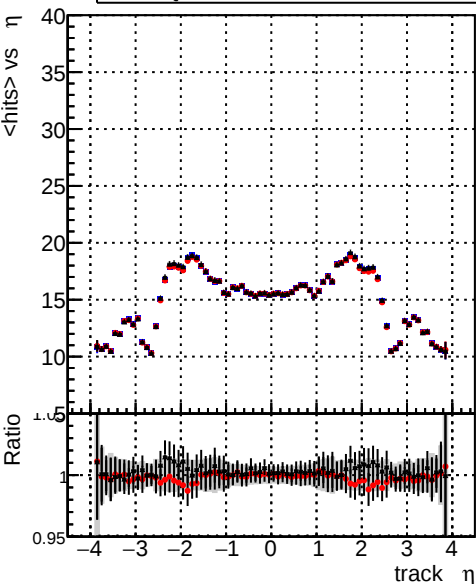
mean hits vs \eta — DQM_test_CKFFitDefault — DQM_test_doubleFit — DQM_test_mkFitFit_noOL
