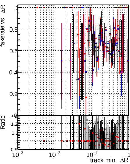
Fake rate vs \Delta R(\text{track, jet}) DQM test CKFitDefault DQM test doubleFit DQM test mkFitFit_noOL
