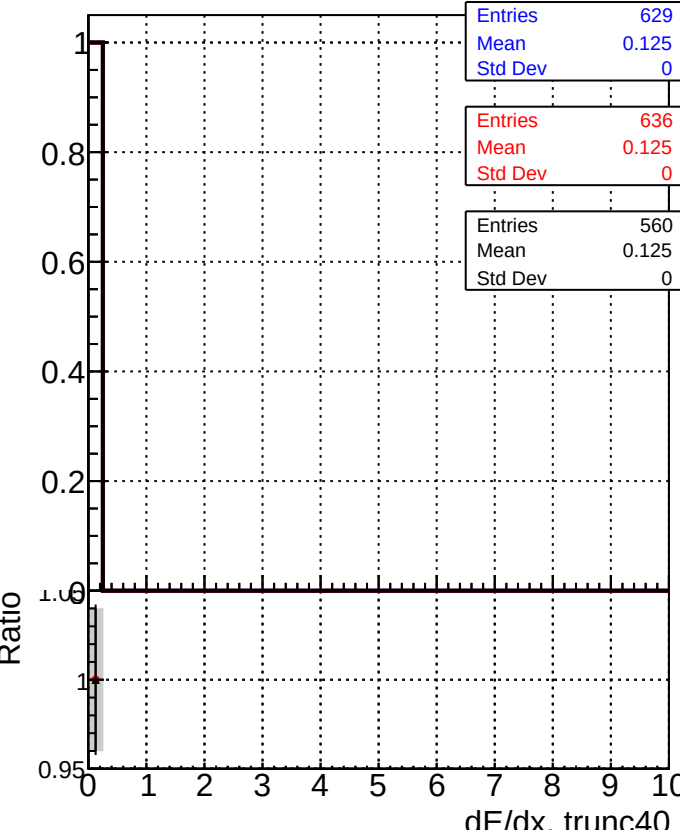
dE/dx estimator 2
