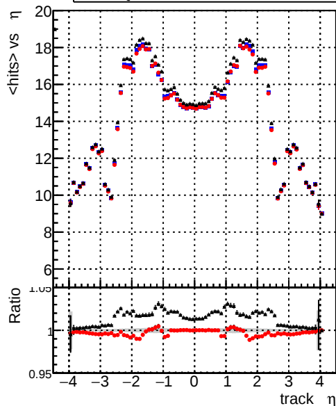
mean hits — DQM_test_CKFFitDefault — DQM_test_doubleFit — DQM_test_mkFitFit_noOL
