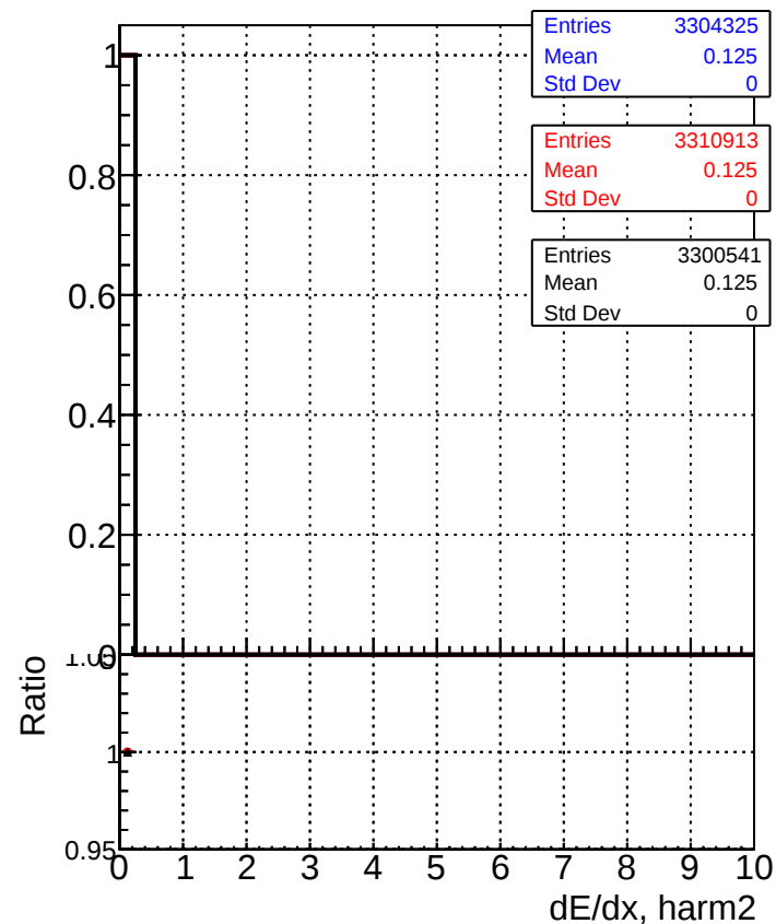
dE/dx estimator 1
