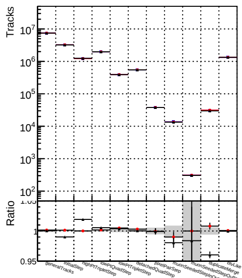
DQM_test_CKFFitDefault DQM_test_doubleFit DQM_test_mkFitFit
