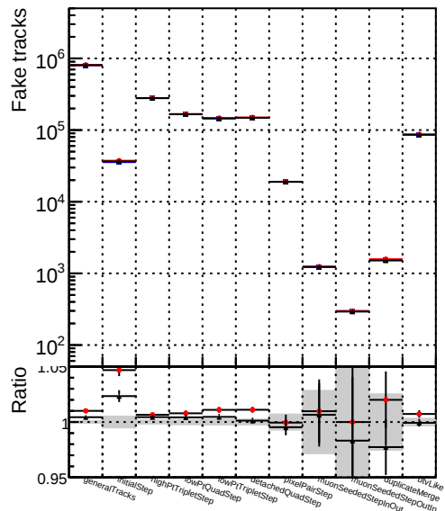
DQM_test_CKFFitDefault DQM_test_doubleFit DQM_test_mkFitFit
