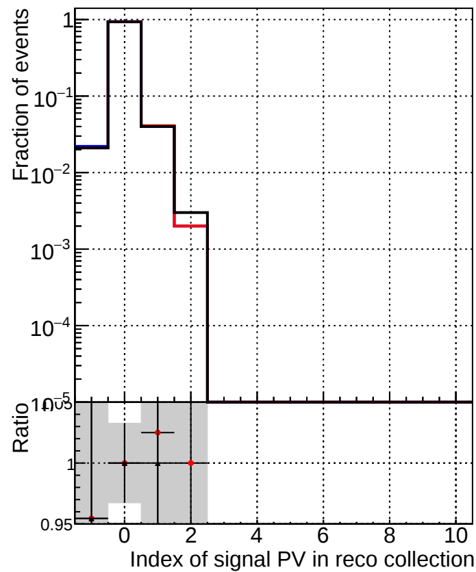
—■ DQM_test_CKFFitDefault —● DQM_test_doubleFit —■ DQM_test_mkFitFit
