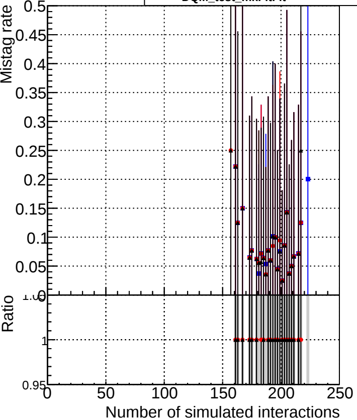
—■ DQM_test_CKFFitDefault —● DQM_test_doubleFit —■ DQM_test_mkFitFit
