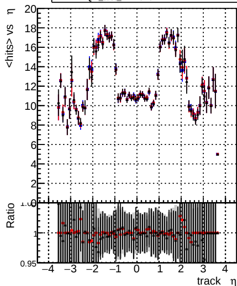
mean hits DQM_test_CKFFitDefault DQM_test_doubleFit DQM_test_mkFitFit
