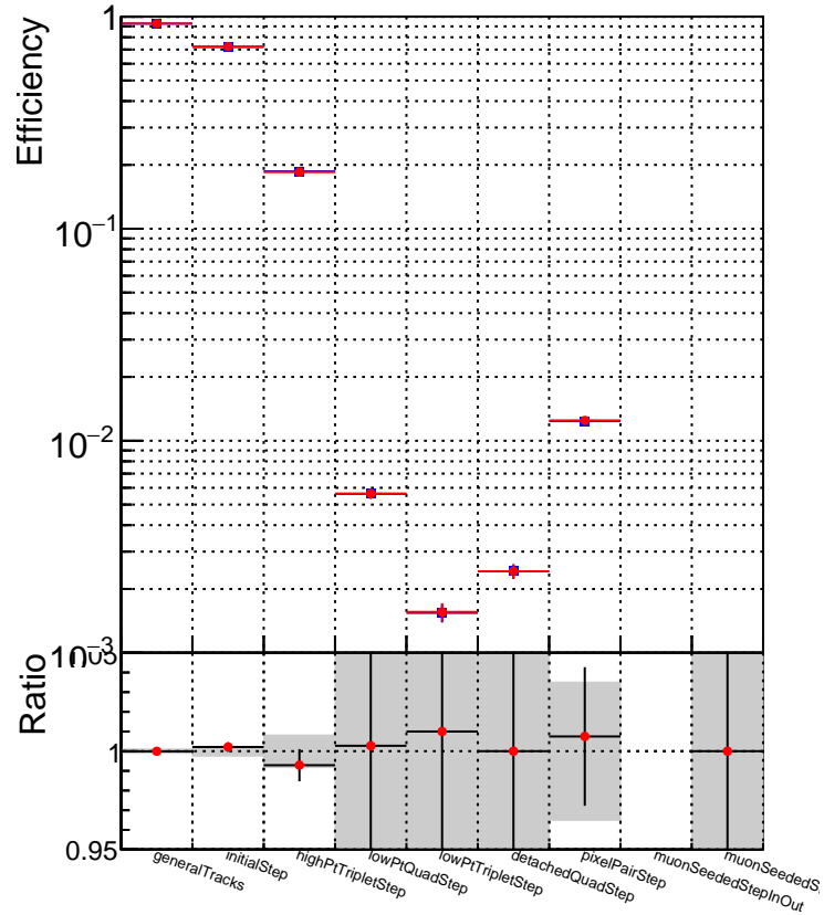
■ DQM_test_CKFFitDefault ● DQM_test_doubleFit
