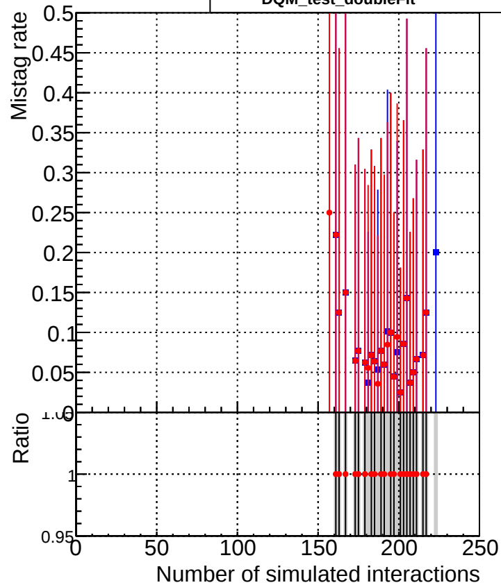
■ DQM_test_CKFFitDefault ● DQM_test_doubleFit
