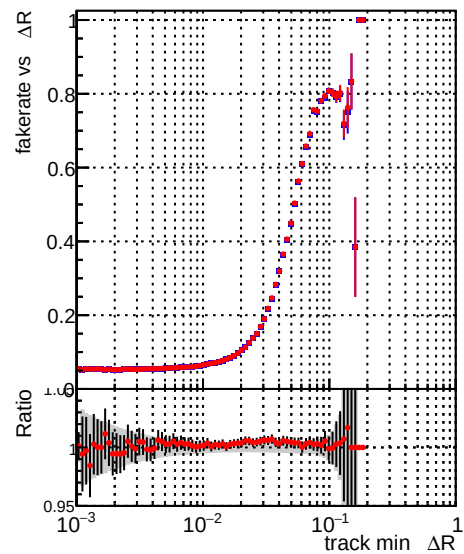
—•— DQM_test_CKFFitDefault —•— DQM_test_doubleFit
