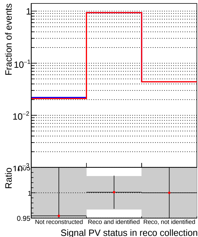
DQM_test_CKFFitDefault DQM_test_doubleFit
