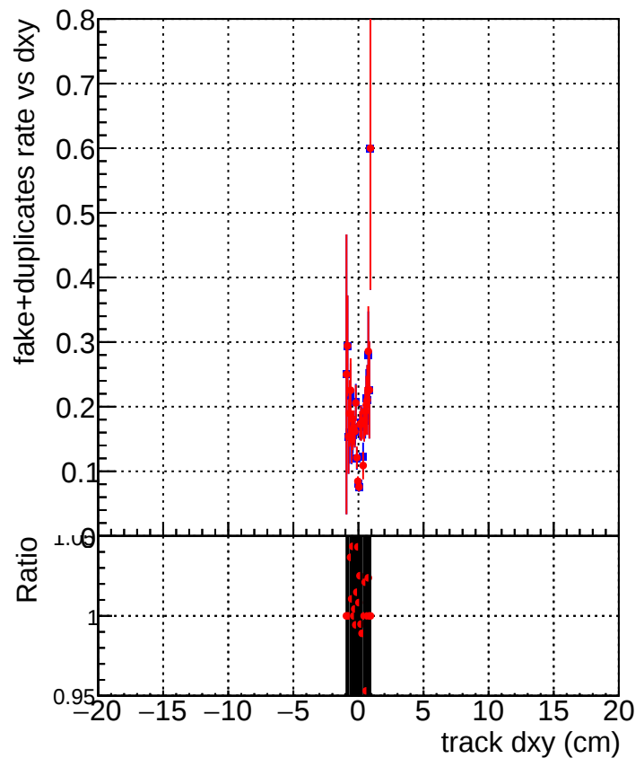
DQM_test_CKFFitDefault DQM_test_doubleFit
