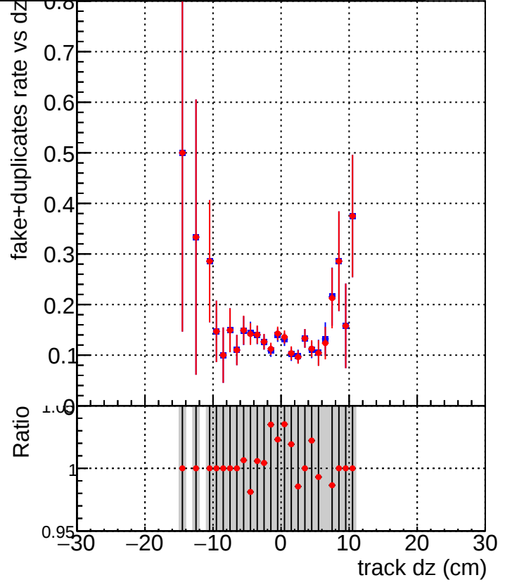
DQM_test_CKFFitDefault DQM_test_doubleFit
