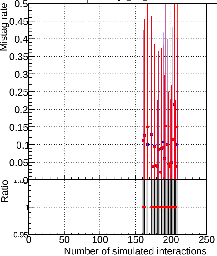
■ DQM_test_CKFFitDefault ● DQM_test_doubleFit
