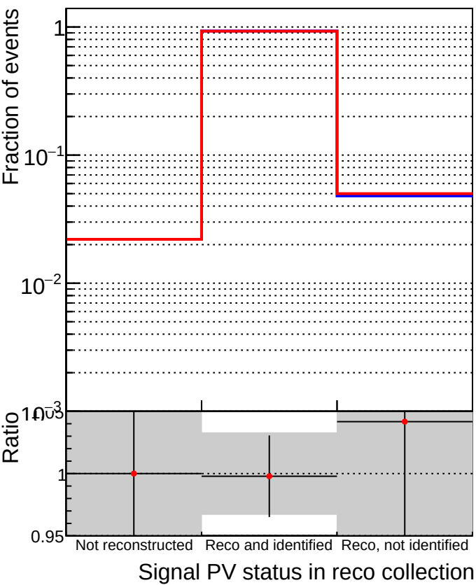
■ DQM_test_CKFFitDefault ● DQM_test_doubleFit
