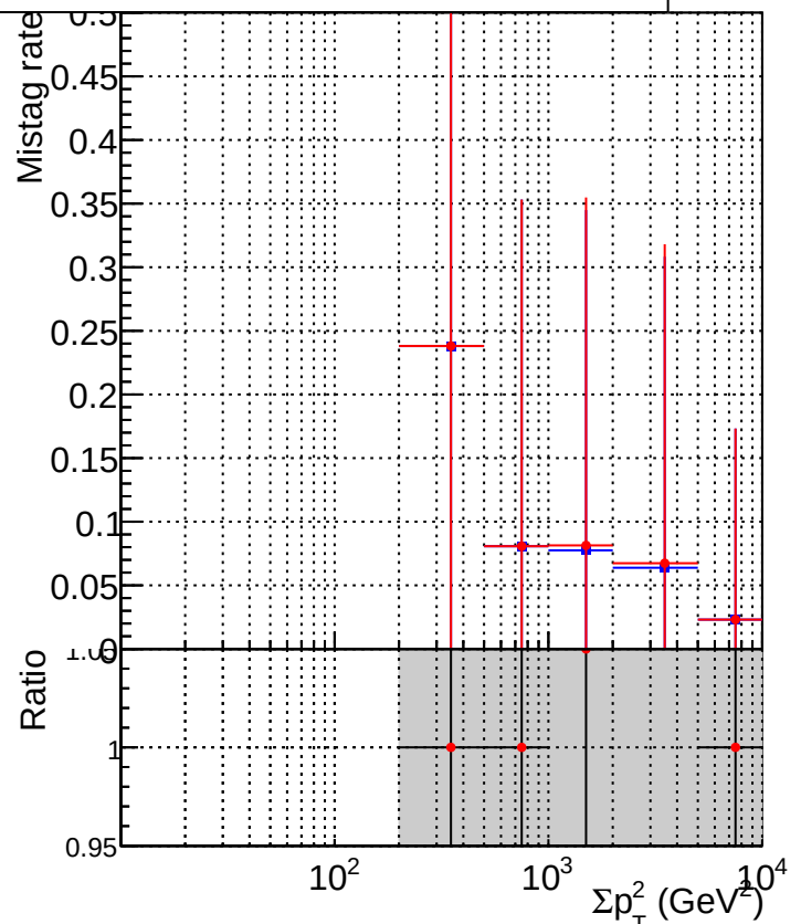
■ DQM_test_CKFFitDefault ● DQM_test_doubleFit
