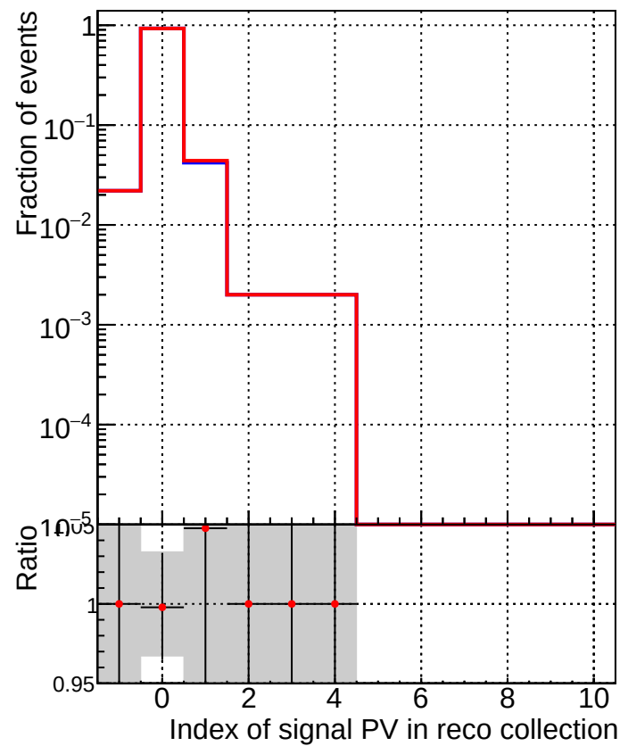
■ DQM_test_CKFFitDefault ● DQM_test_doubleFit
