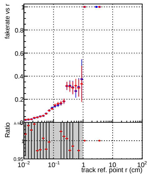
—■— DQM_test_CKFFitDefault —●— DQM_test_doubleFit
