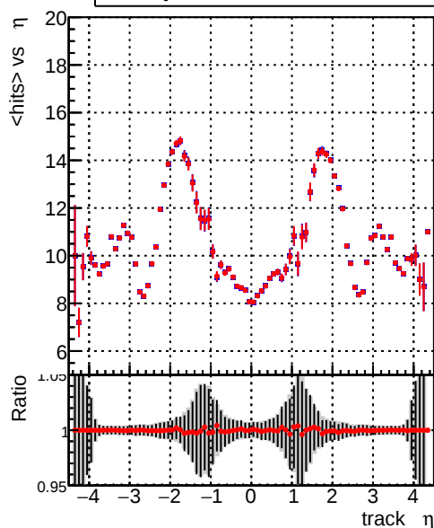
mean hits — DQM_test_CKFFitDefault — DQM_test_doubleFit
